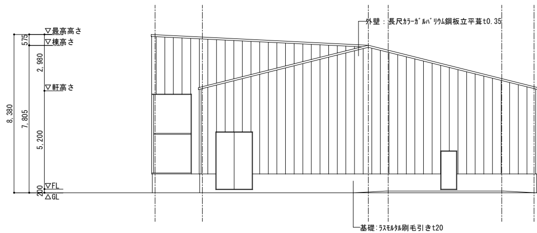
北面立面图
