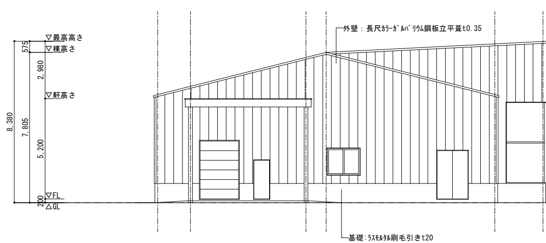
南面立面图
