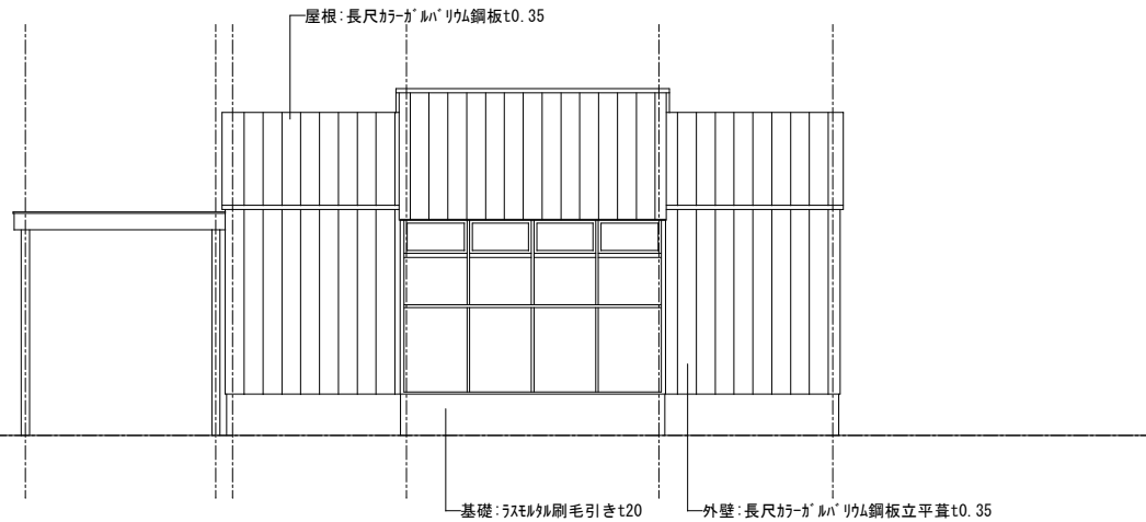
東面立面图
