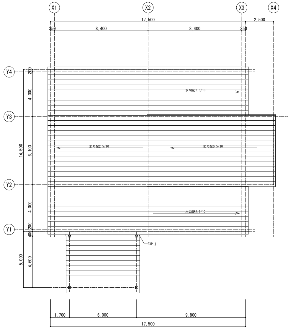
屋根伏図
