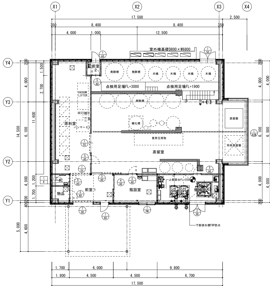
1 階平面図
