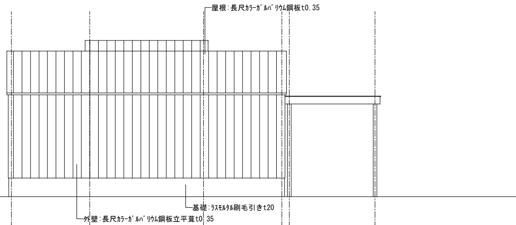
西面立面图
